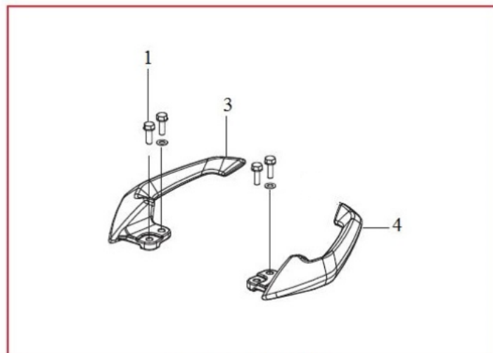
ALÇA TRASEIRA
