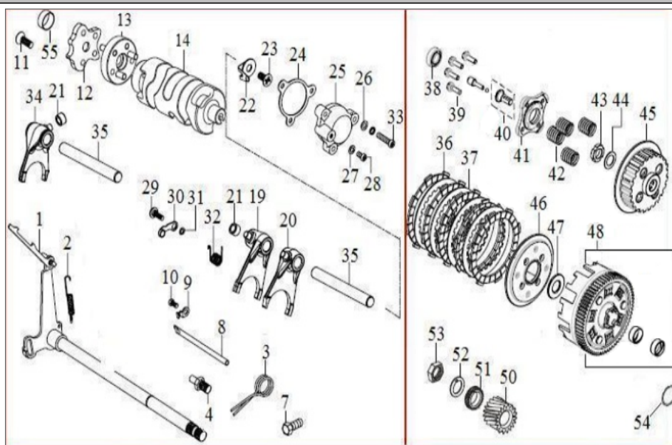
TAMBOR SELETOR
