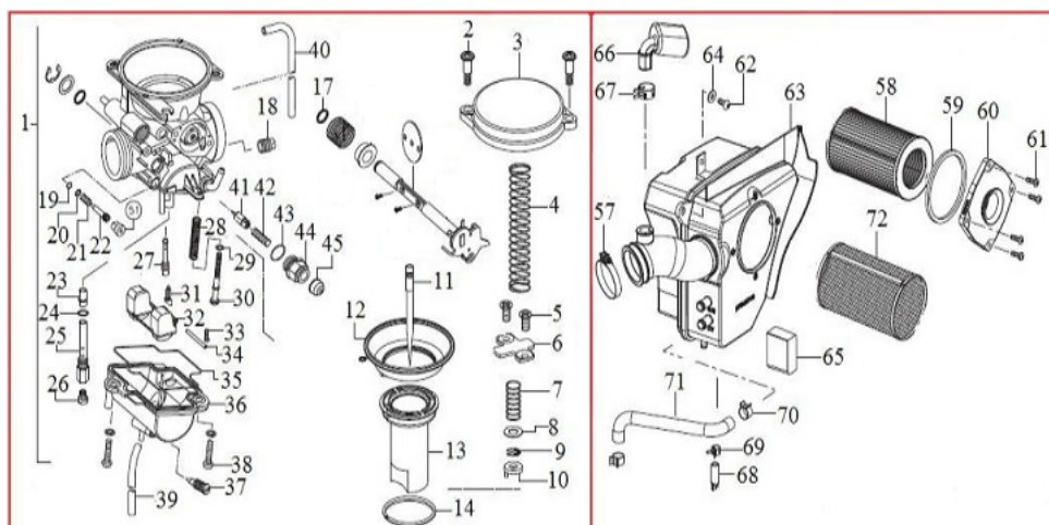
CARBURADOR
