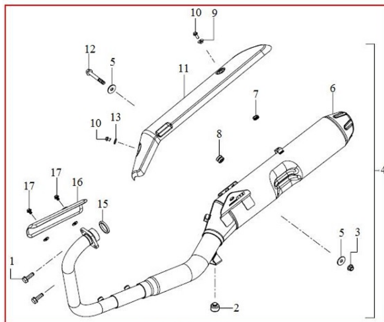
ESCAPAMENTO
