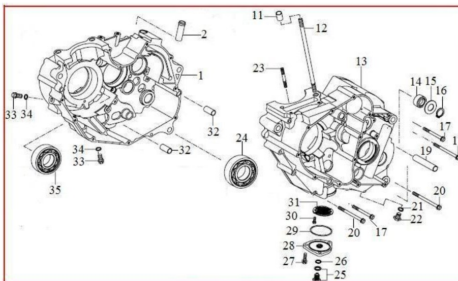
CARCAÇAS
