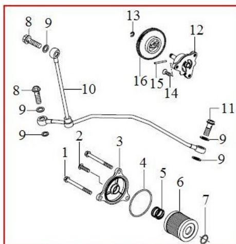
BOMBA / FILTRO DE ÓLEO
