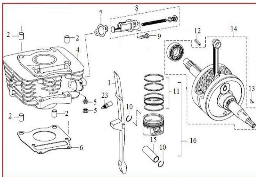
CILINDRO, VIRABREQUIM E PISTÃO
